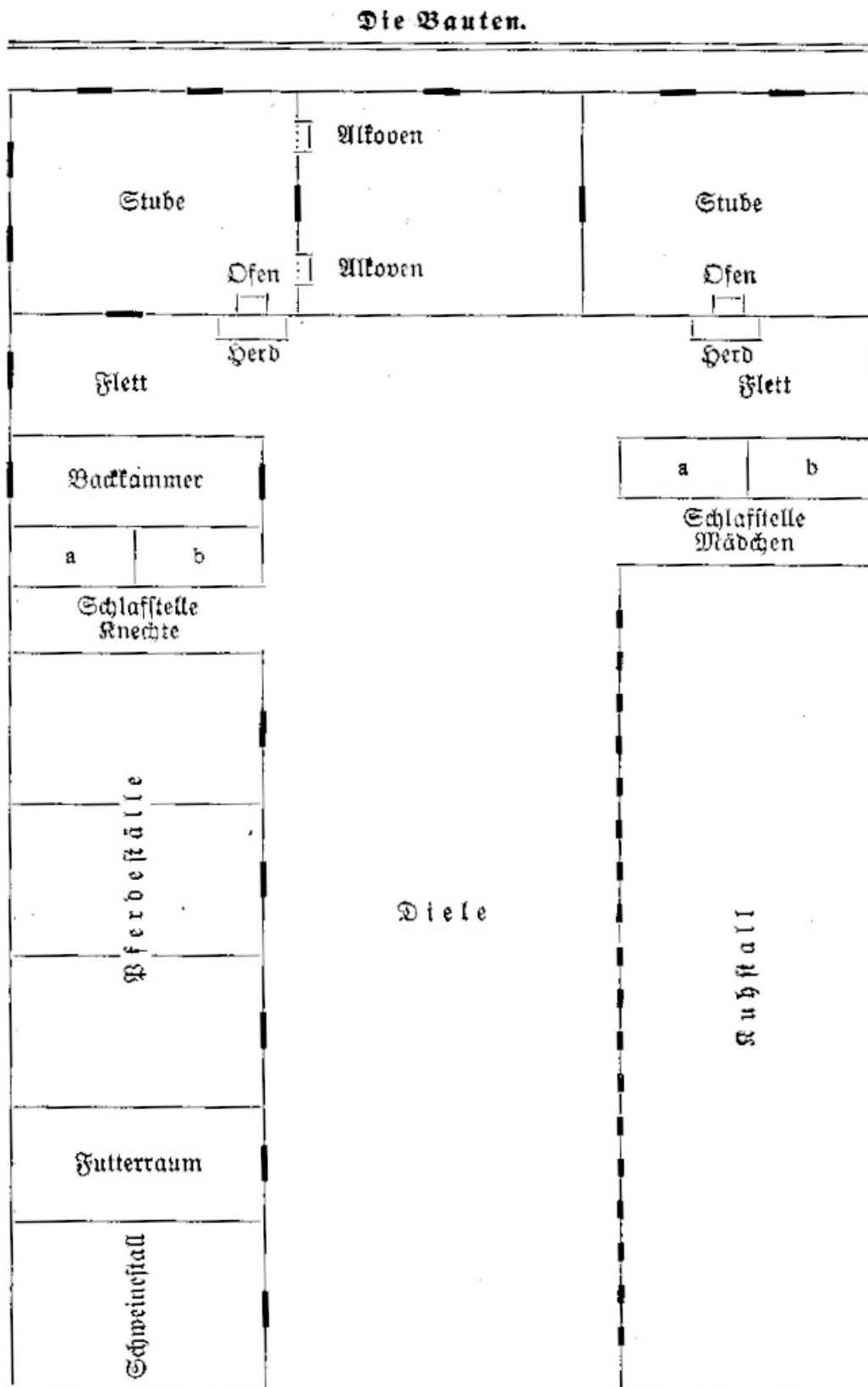
Grundriß vom Sachsenhaus (Einhaus).
